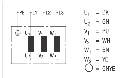
Star (3~ 400 VAC)
