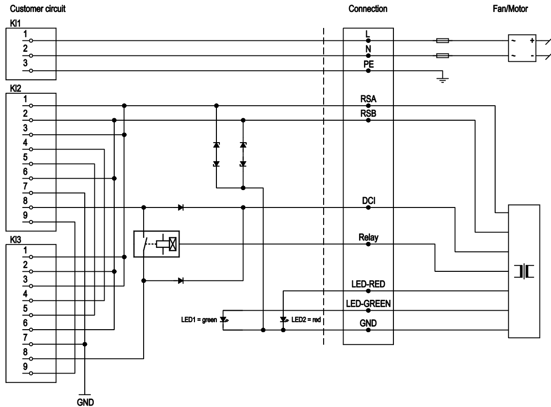
LED1 / LED2
