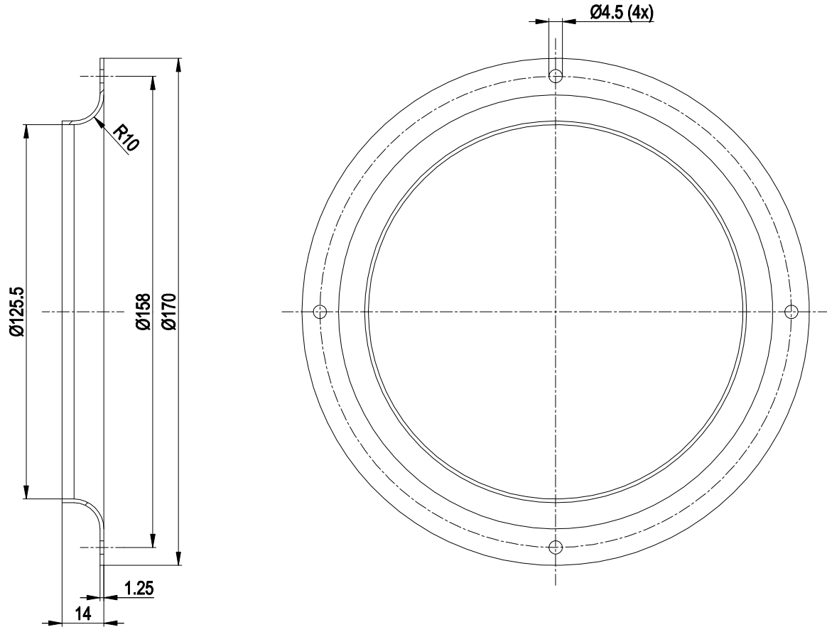
Inlet ring 09576-2-4013
