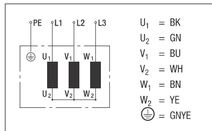
Star (3~ 400 VAC)
