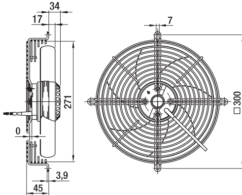
Delta (3~ 230 VAC)
