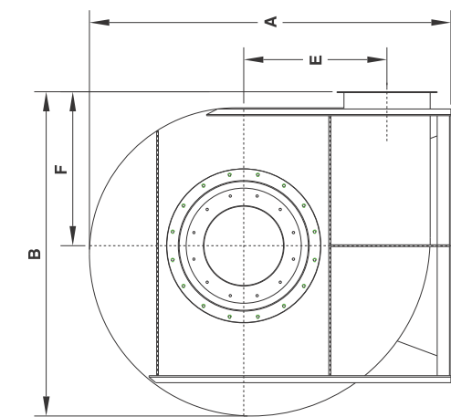
APRGc 1251...1801
